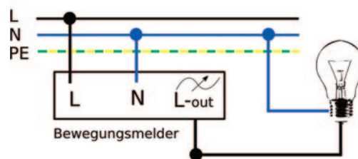
Anschlussbild 3-Draht Bewegungsmelder
